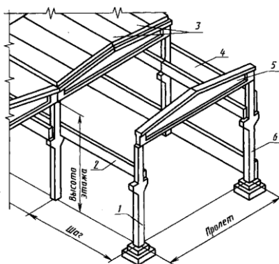
Рисунок 1 - Конструктивные элементы здания
